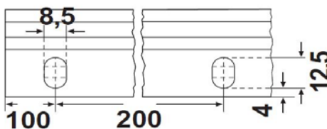
Standardní vrtání pro C-14 a C-15 / Standard drilling for C-14 and C-15
