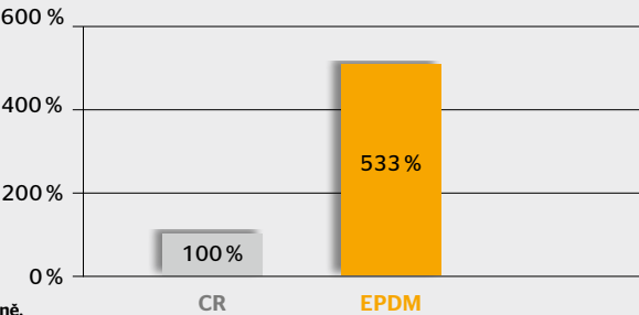
Test životnosti při 120 °C okolní teploty**
